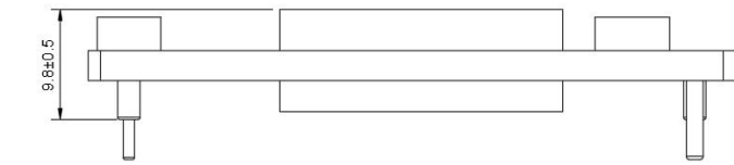
标准型 58.1mm*23.0mm*9.8mm
